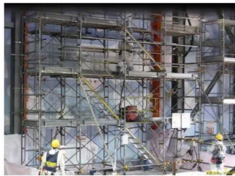
調査用コア採取の作業状況(全景)
