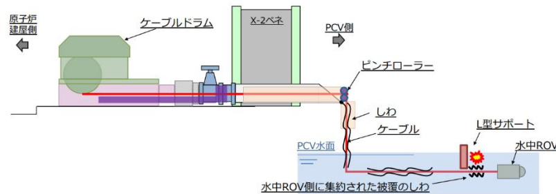
図1.水が浸入した推定原因（イメージ図）
