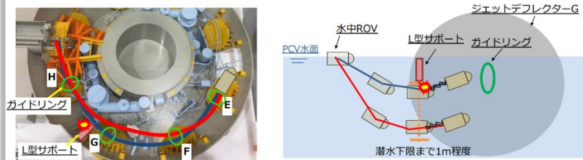
図1.水平方向での回避対策（イメージ図）
