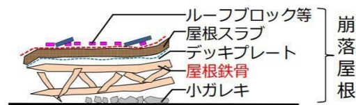
図2 崩落屋根の状態
