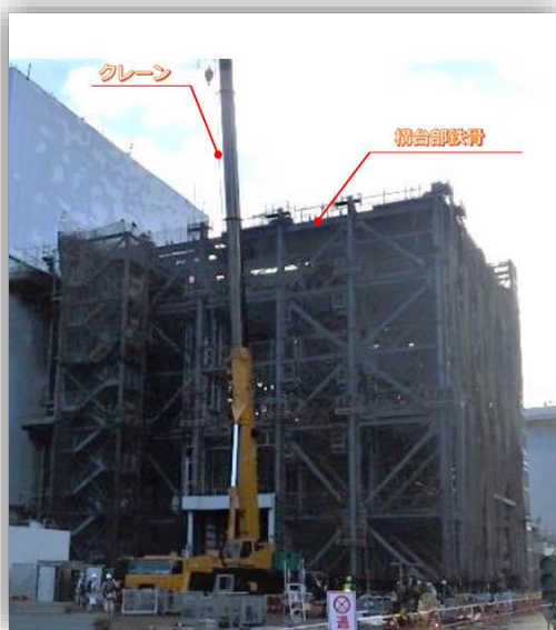
（組み立てが完了した構台の鉄骨ユニット）
