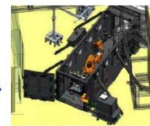
ハッチ開放装置の 隔離部屋③への搬入
