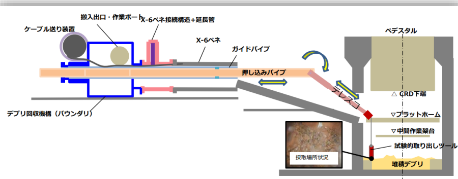
テレスコ式装置のイメージ図
