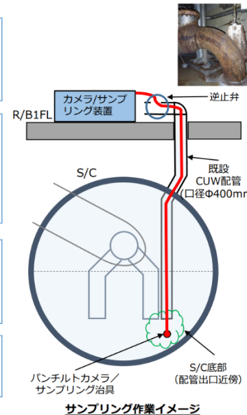
(S/C内包水サンプリング作業ステップ)
