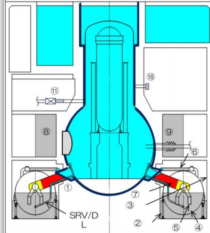
図 燃料取出しのためのPCV冠水範囲構成 (ウェル満水とした場合) (1F-1号機/2, 3号機)
