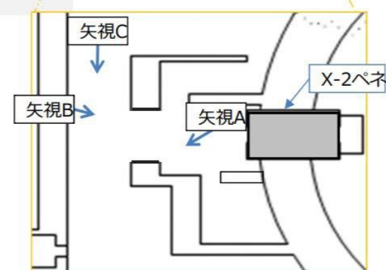
1号機原子炉建屋1階
