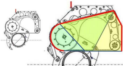
飛散防止カバー取付イメージ
