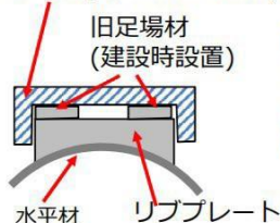
図1 足場断面図
