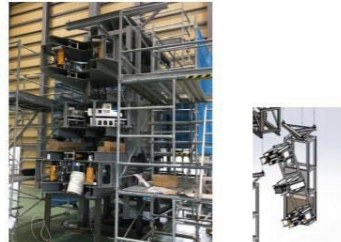
鉄塔解体装置（斜材用）組立状況
