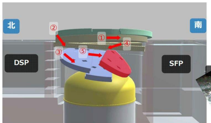
ウェルプラグイメージ図 (西側)
