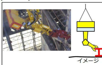
図4 カッター (当初計画)
