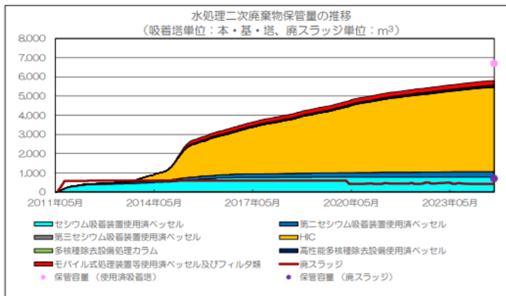
水処理二次廃棄物の管理状況(2024.10.3時点)
