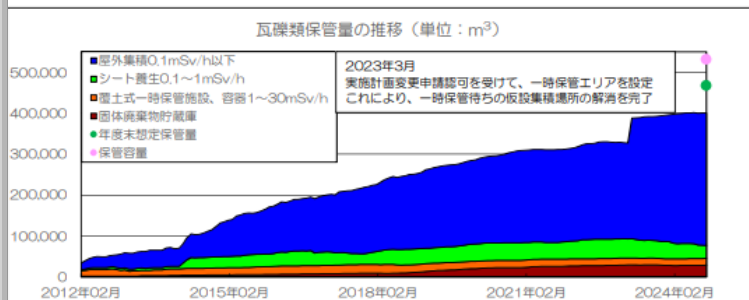
瓦礫類・伐採木・使用済保護衣等の管理状況(2024.9.30時点)
