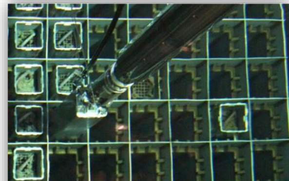
共用プール燃料ラックへの収納
