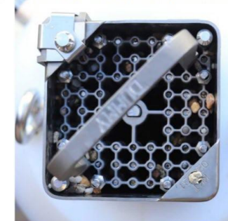
試験後燃料集合体上部 (ダミー燃料)
