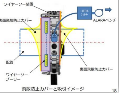
飛散防止カバーと吸引イメージ
