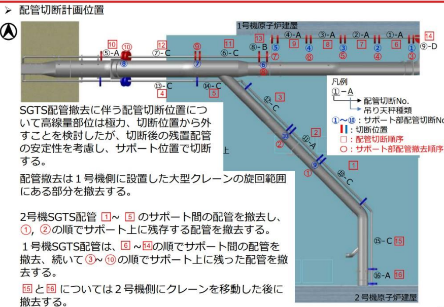
【参考】発泡ウレタン注入後の切断順序 (2号機⇒1号機)
