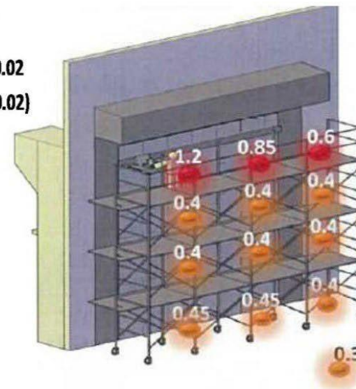
西側外壁面
