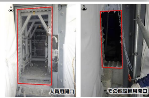
写真②：人員用及びその他設備用開口設置状況 (撮影日：2024.12.13) 南側構台側より撮影
