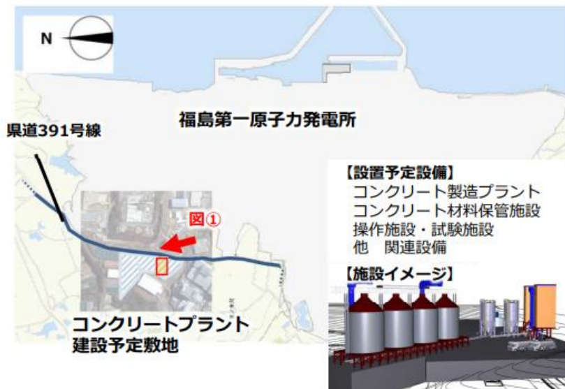
敷地配置図
