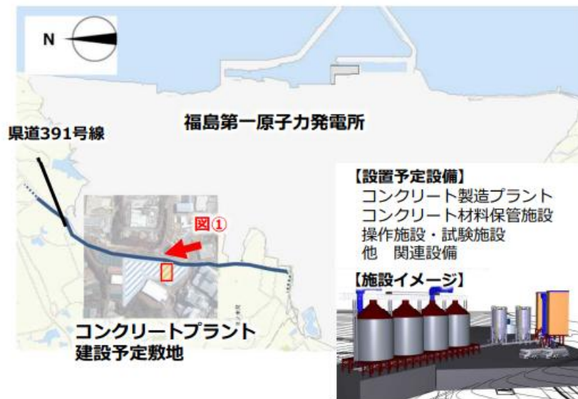
敷地配置図
