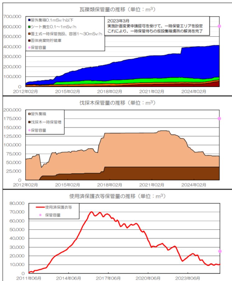
瓦礫類・伐採木・使用済保護衣等の管理状況(2025.11.30時点)
