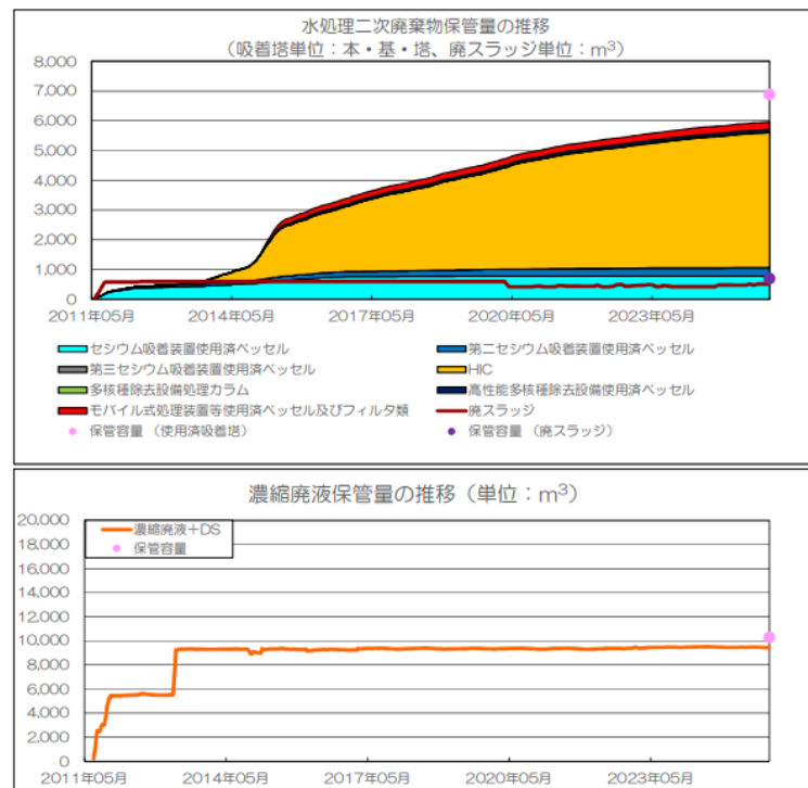
水処理二次廃棄物の管理状況(2025.12.4時点)
