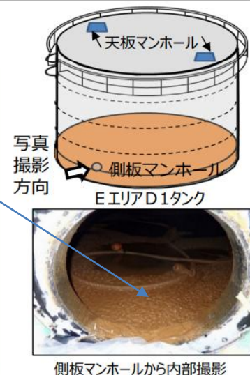
側板マンホールから内部撮影
