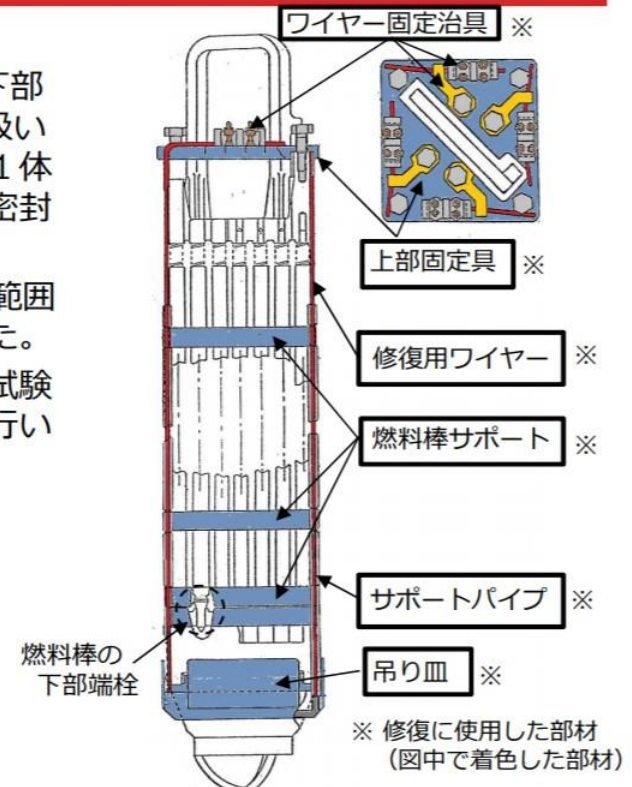
ワイヤー修復燃料のイメージ図
