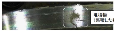
キャスクフランジ面 (清掃時に堆積物を集積した状態)
