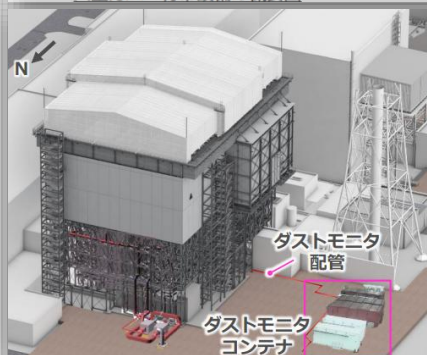
大型カバー付帯設備の概要図
