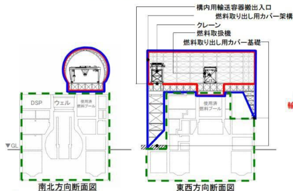
3号機燃料取り出し用カバー 完成イメージ
