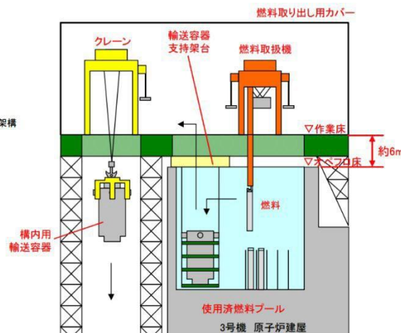
3号機燃料取り出し作業イメージ
