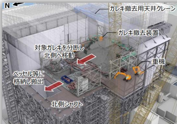
ガレキ撤去のイメージ
