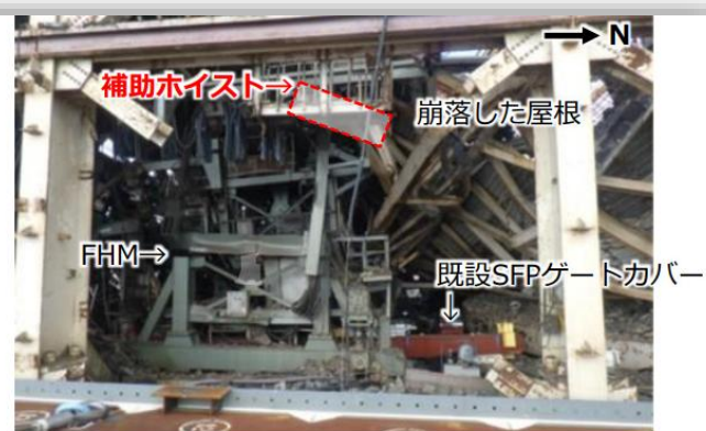
1号機オペフ口面を東から見た写真
