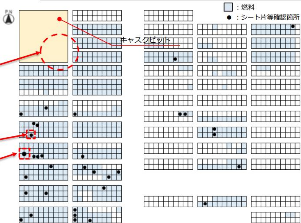
2号機使用済み燃料プール内の状況
