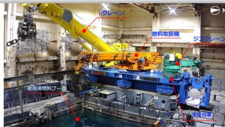
原子炉建屋内燃料取扱設備全景(遠隔監視カメラにて撮影) (撮影：2025年12月6日)
