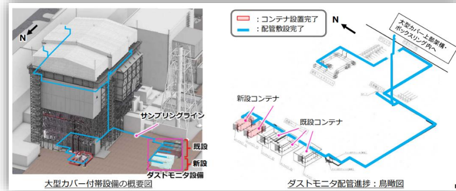
大型カバー付帯設備の概要図
