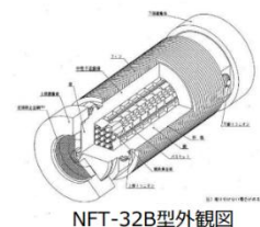
NFT-32B型外観図
