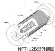
NFT-12B型外観図
