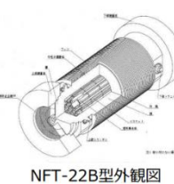
NFT-22B型外観図
