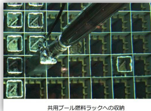
共用プール燃料ラックへの収納
