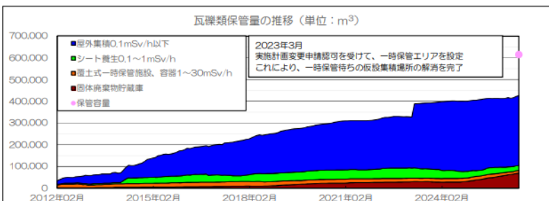
瓦礫類・伐採木・使用済保護衣等の管理状況(2026.6.30時点)
