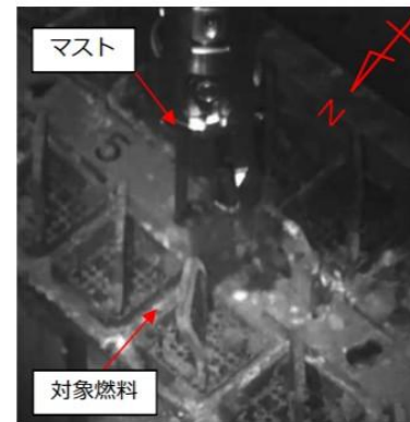
マスト 対象燃料 マストと配管の干渉により 吊ることができない燃料 (No.⑭※)
