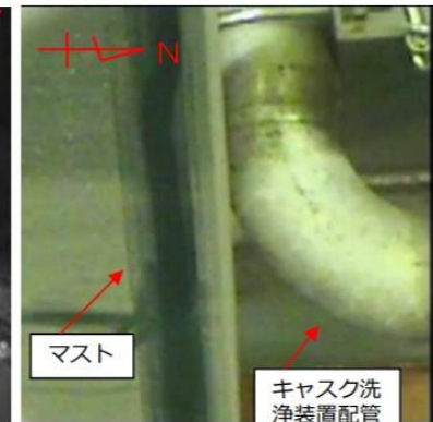
マスト キヤスク洗 浄装置配管 マストとの干渉の状況(No.⑭※)
