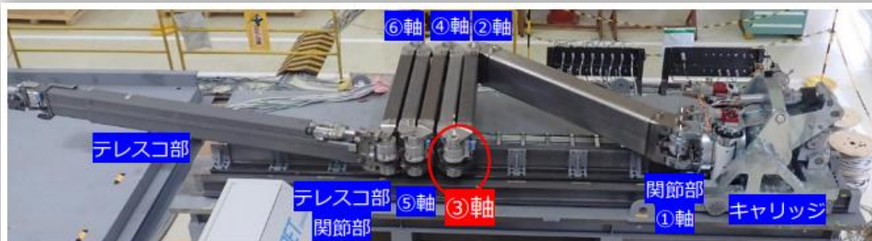
ロボットアーム概要
