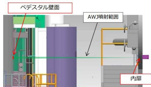
X-2ペネ前断面図 (PCV内)
