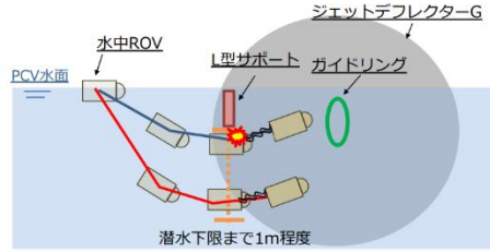
図2. 垂直方向での回避対策（イメージ図）
