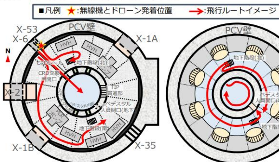
3号機 D/W 1FL 平面概略図
