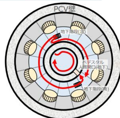
3号機 D/W B1 平面概略図
