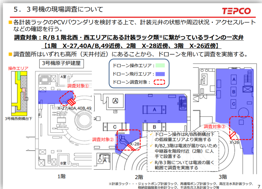
(3号機調査箇所平面図)
