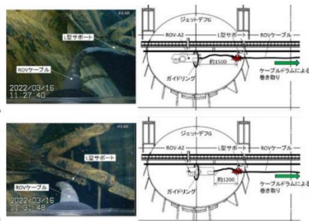
写真2. ケーブル被覆がL型サポートに掛かっている状況
