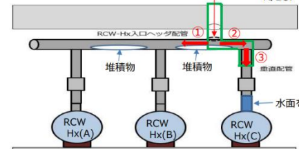
②RCW-H(C)側の配管底部の堆積物
