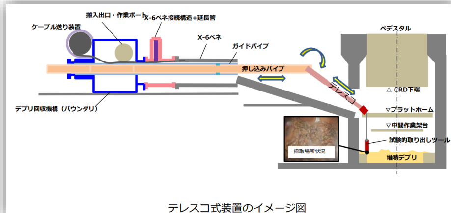
テレスコ式装置のイメージ図
