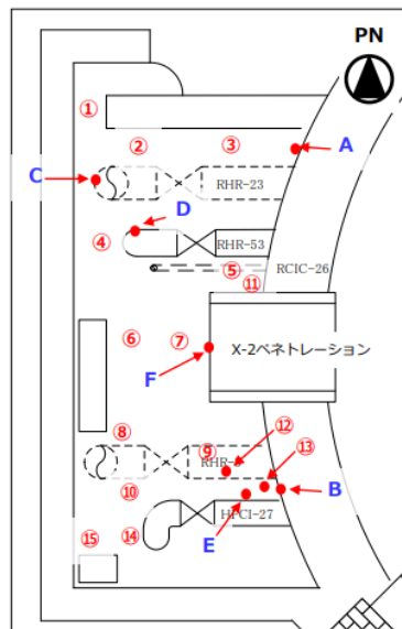
P/A室 線量測定位置
