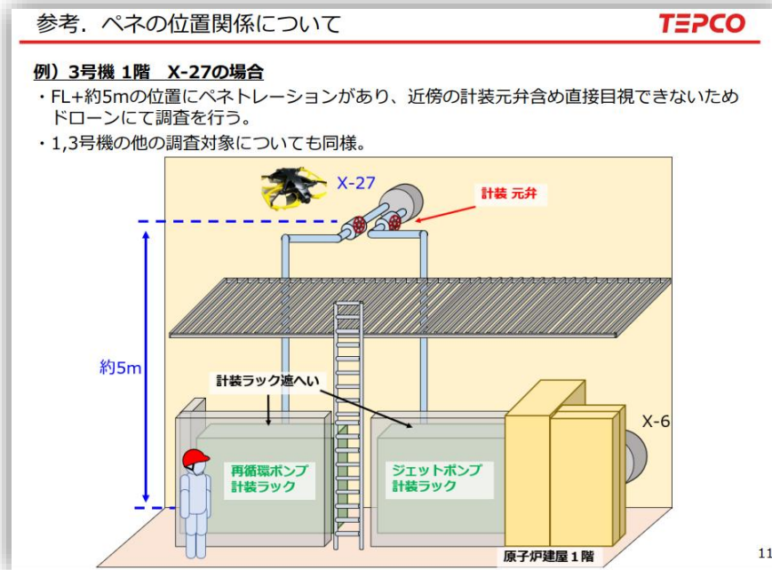
(3号機調査箇所立面図)
