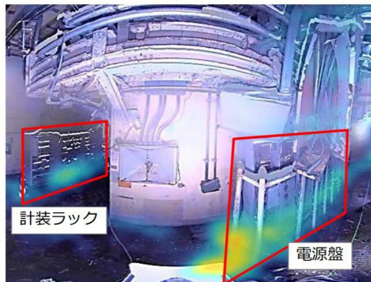
計装ラックおよび電源盤の線源 (ガンマカメラ画像)
