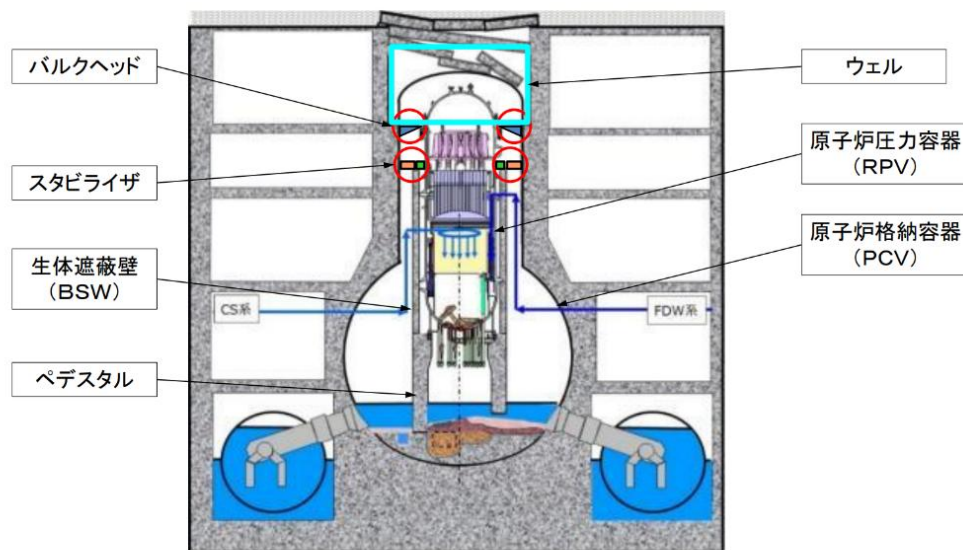
図2-① 1号機構造物配置概要
