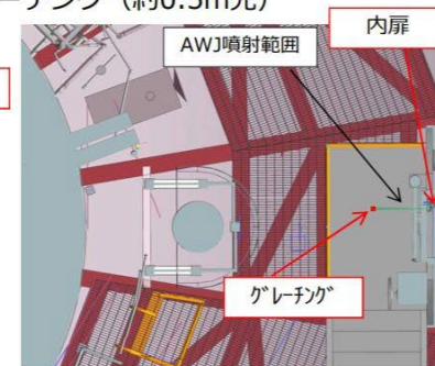
X-2ペネ前水平面図 (PCV内)
