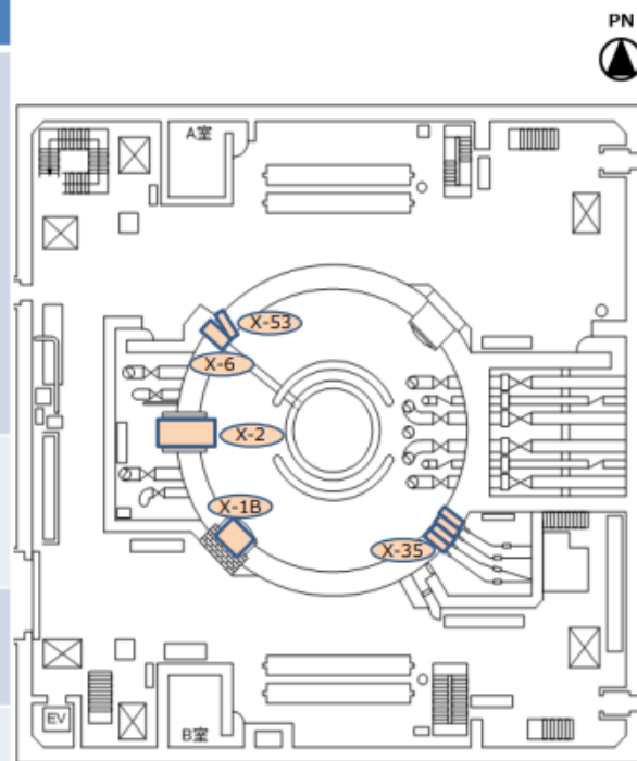
3号機原子炉建屋1階
