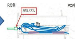
堆積物除去装置 (高圧水、AWJ)
