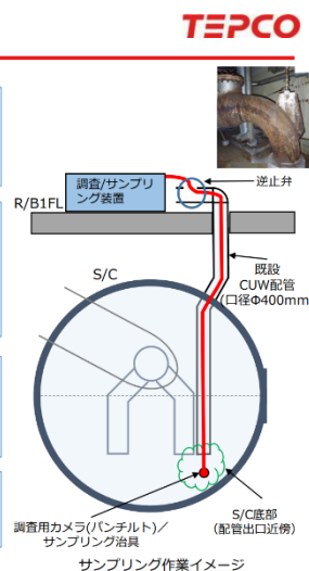
サンプリング作業イメージ
