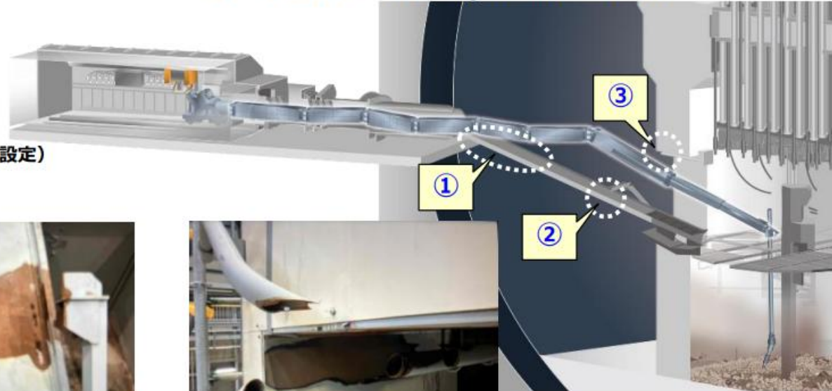
② CRDレール吊り治具
