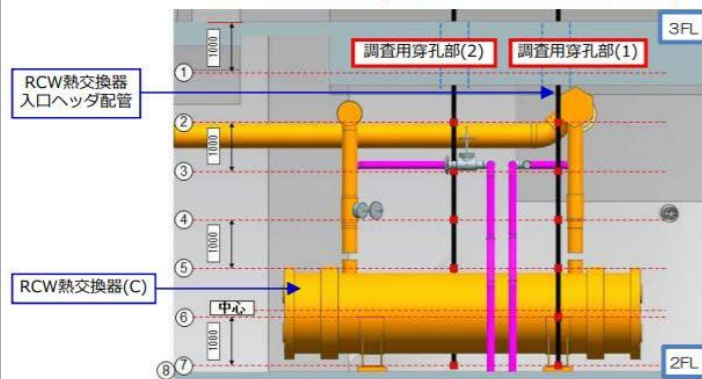
線量測定位置(3階-2階断面図)
