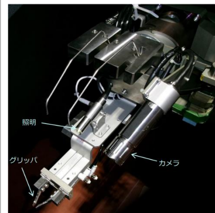
グリップパ型 グリップパ方式先端治具
