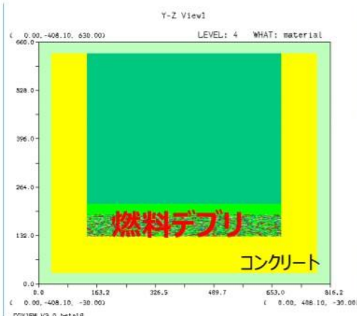
計算モデル
