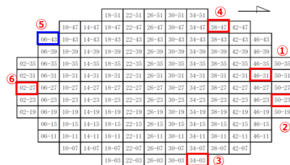
CRDロケーション図 (原子炉底部)
