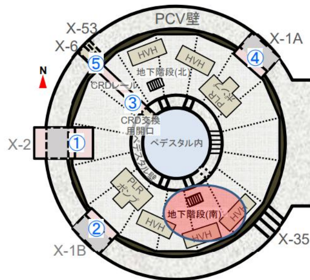
3号機D/W1FL 平面概略図
