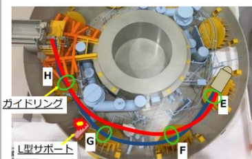
図1. 水平方向での回避対策（イメージ図）
