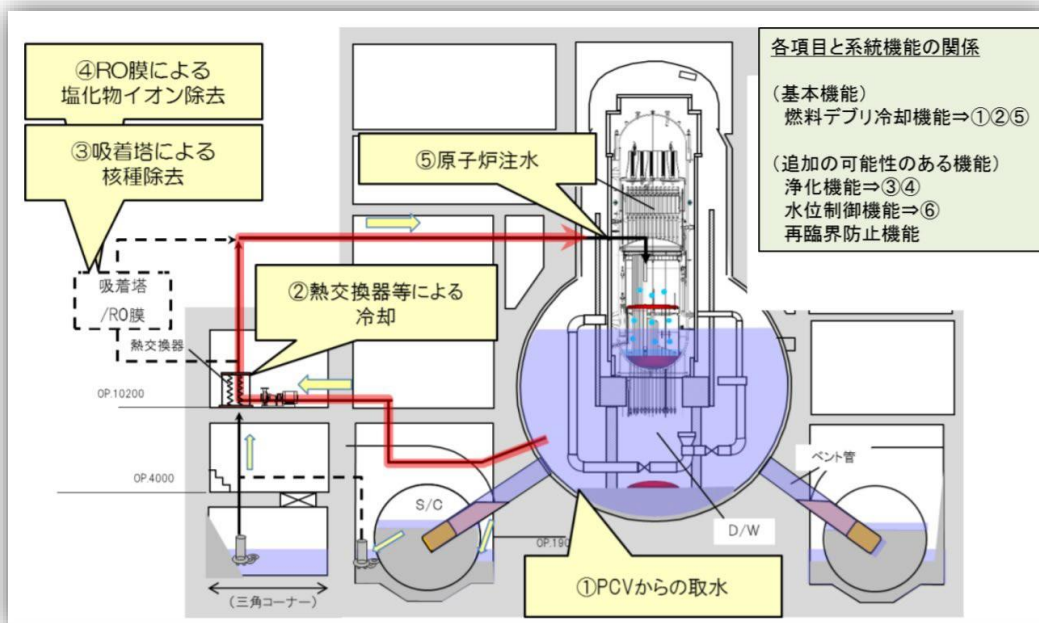
(格納容器循環注水冷却システム概要図)
