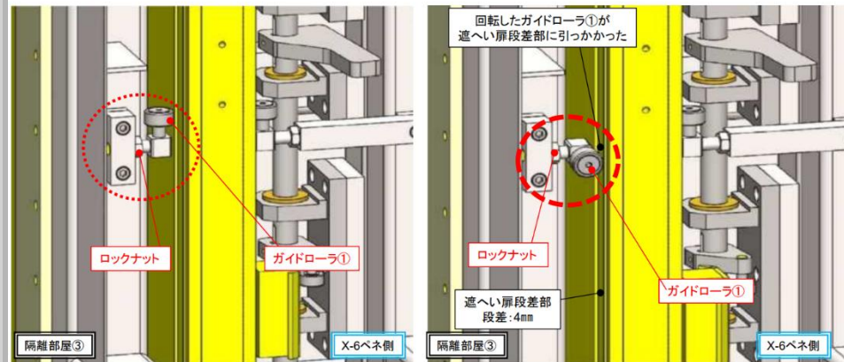
ロックナット通常設置状態
