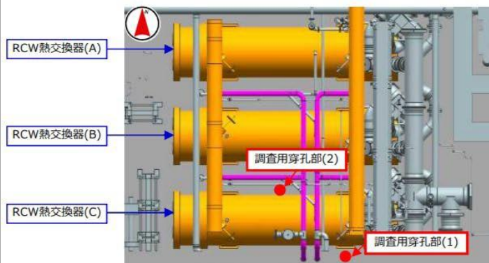
線量測定位置(3階からみた2階平面図)
