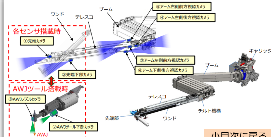
ロボットアーム搭載カメラの状況
