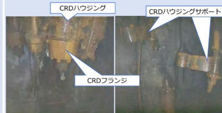
CRD関連機器の状況(左：ハウジング、右：サポート)
