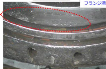
フランジ清掃後
